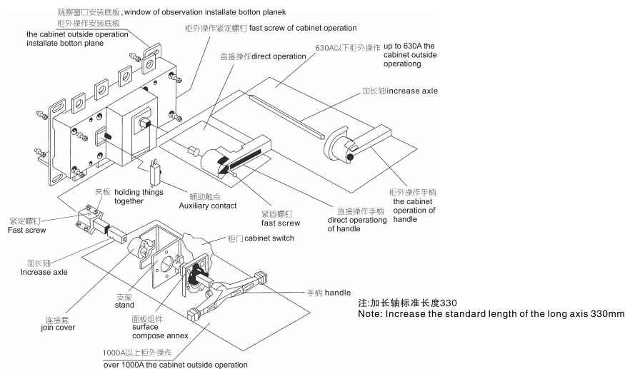
图1 GSG2-160~1600隔离开关
