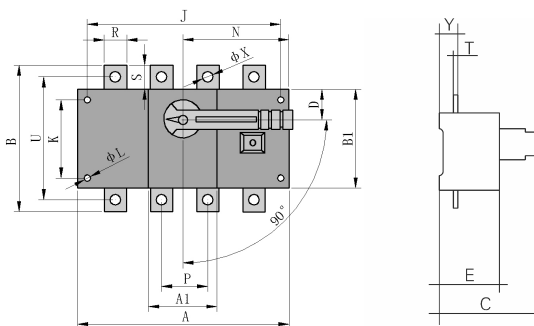
GSG2-160~630柜内操作
