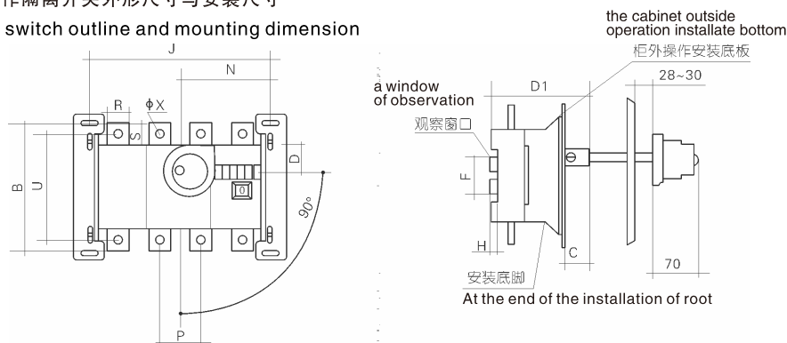
GSG2-160~630/JKH柜外操作
