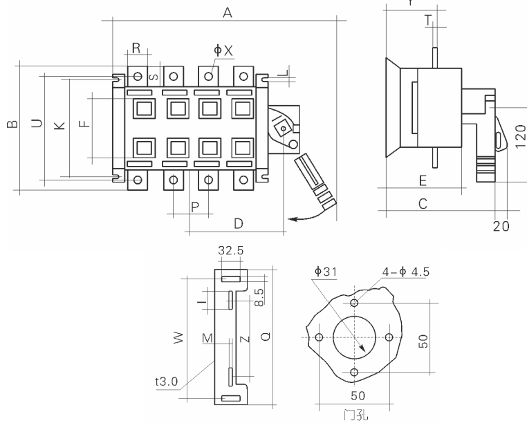
柜外操作安装底板尺寸 (需要特殊定制)
